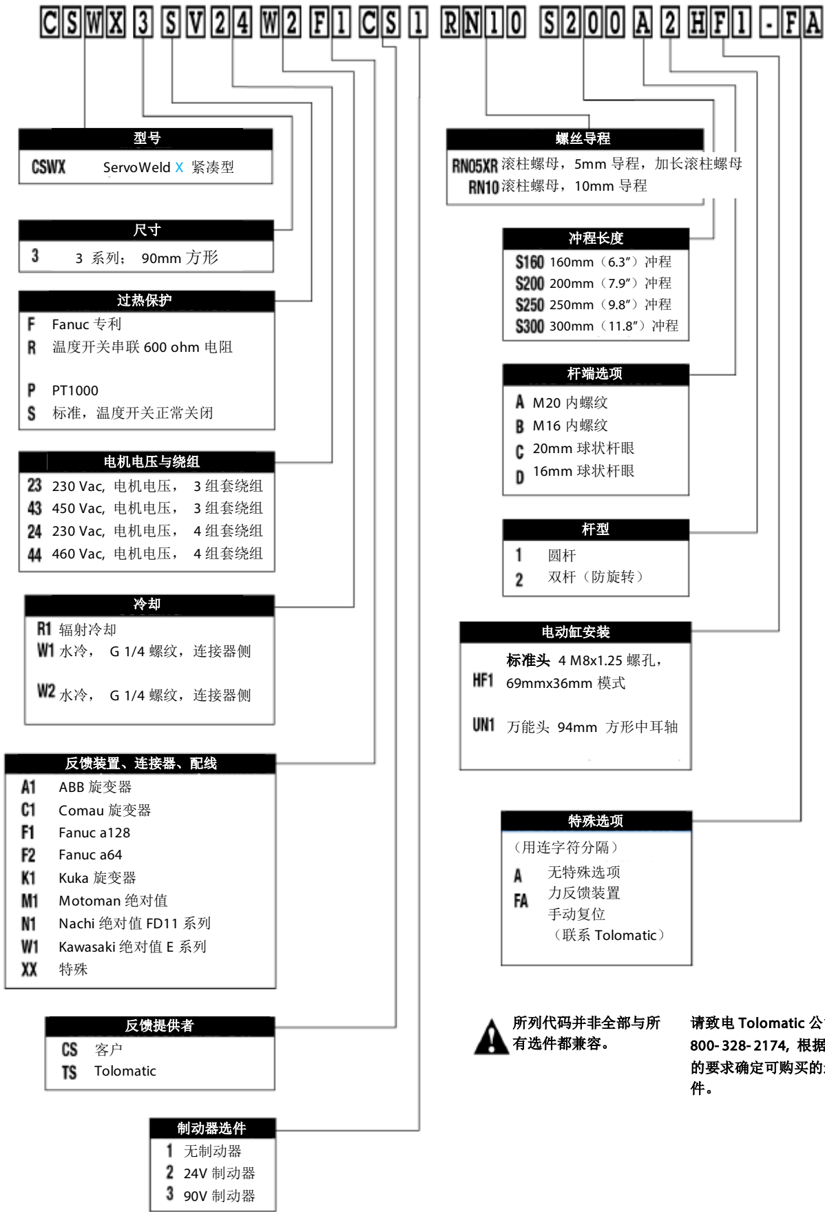
图 3.1 CSWX 订购代码及说明
