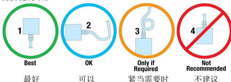
图 5.1: 推荐的 ServoWeld 布线路由。
